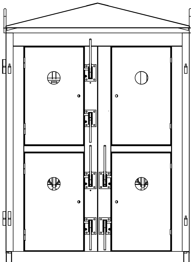
Вид со стороны РУВН (ворота не показаны)
