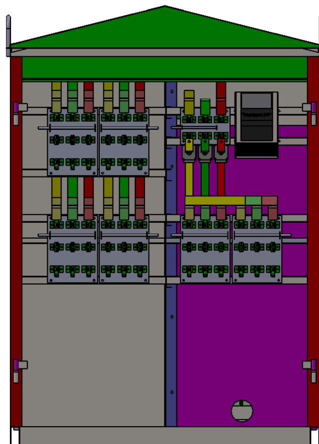
Ошиновка РУНН Вид спереди (передняя панель не показана)
